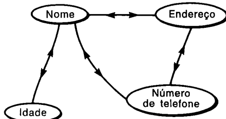
Figura 5.6 Armazenamento relacional
